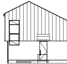
東立面図
