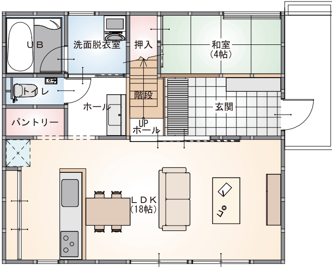
1階平面図
