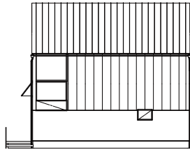
北立面図
