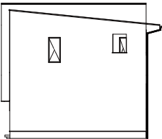
西立面図
